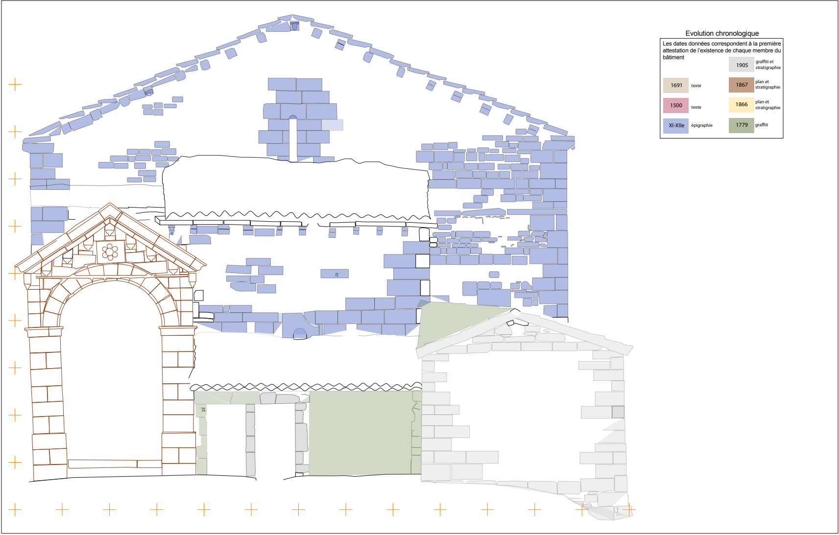
Façade est, phasage chronologique de l'élévation
