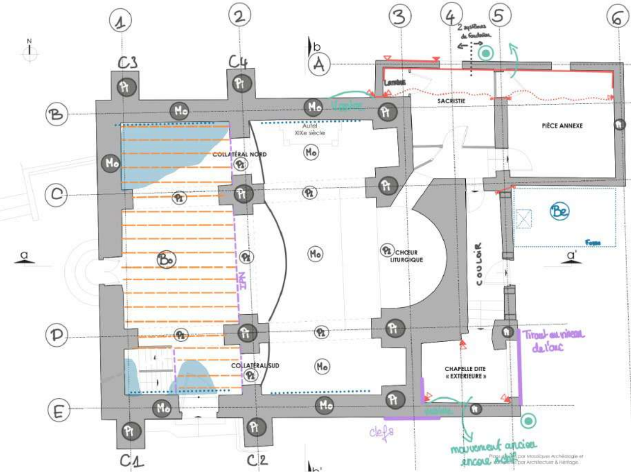
Fig 31. Plan de la chapelle ©EQ
