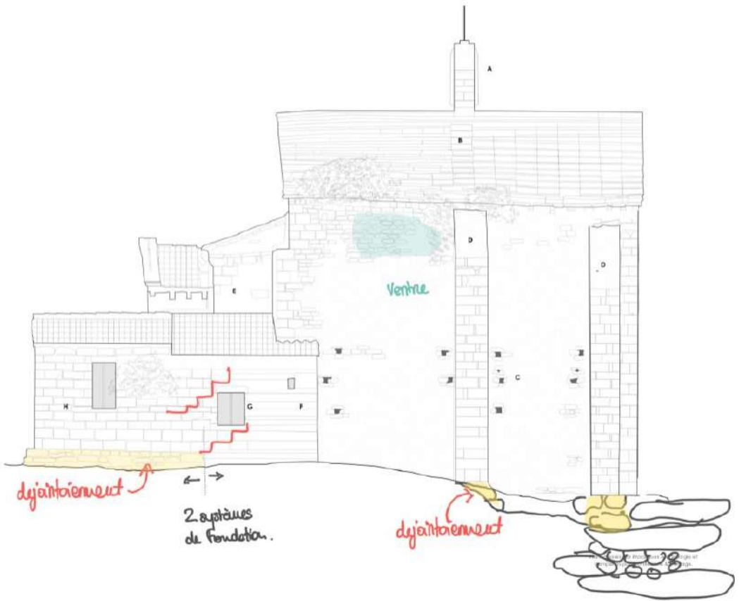
Fig 33. Façade Nord ©EQ
