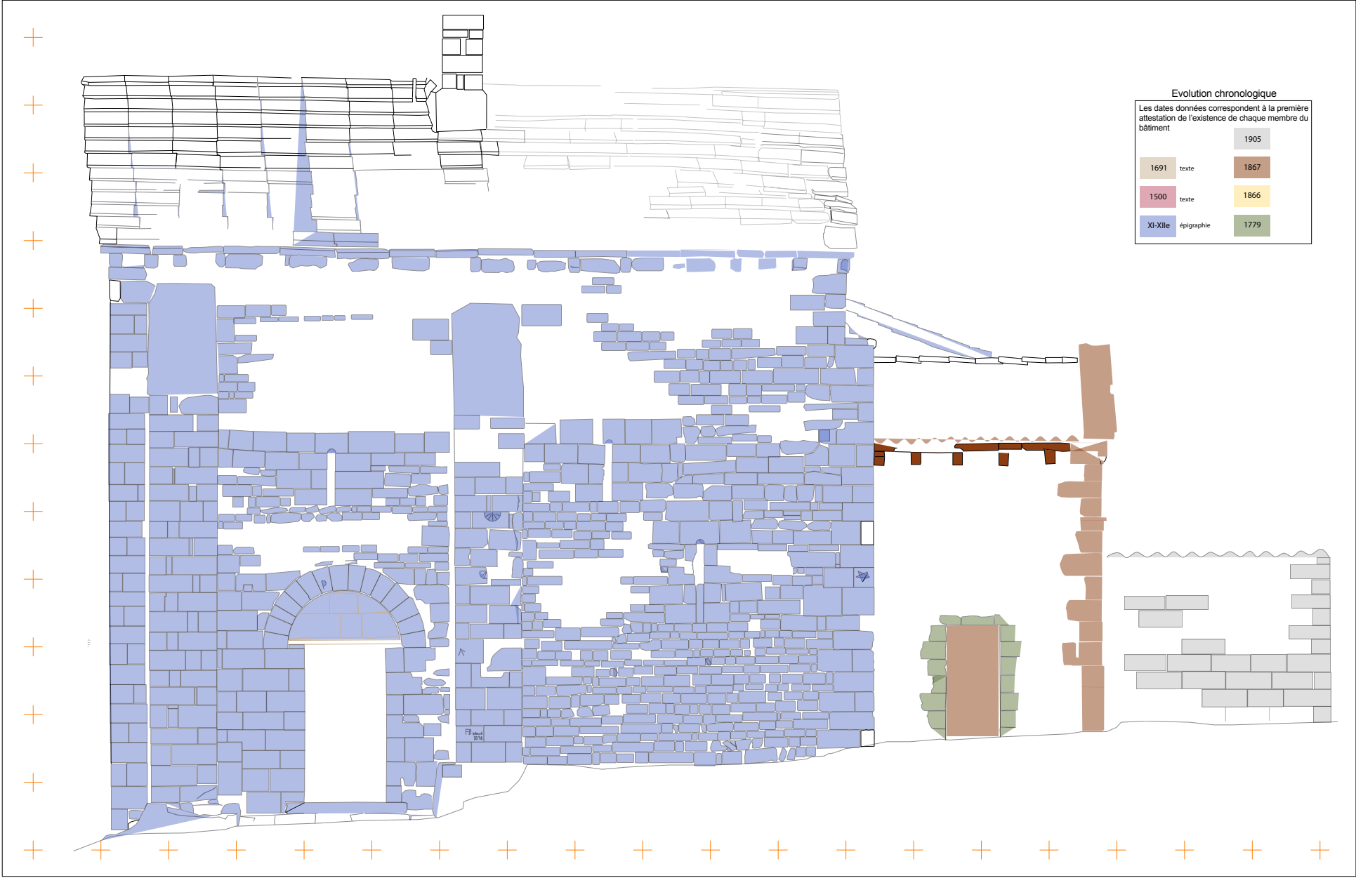
Façade sud, phasage chronologique de l'élévation
