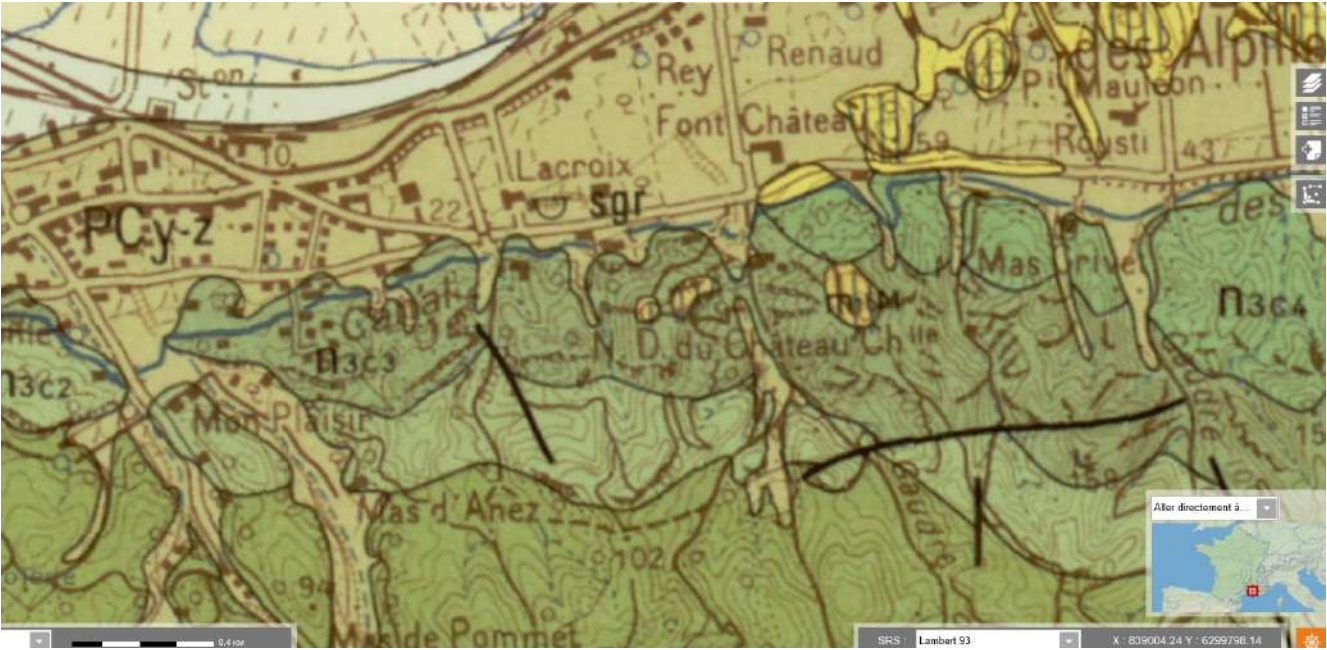
Extrait de la carte géologique, Infoterre. En jaune les gisements de mollasse miocène.
