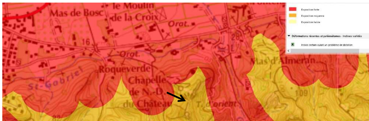
Fig 3. Aléa Retrait-Gonflement des sols ©BRGM BSS
